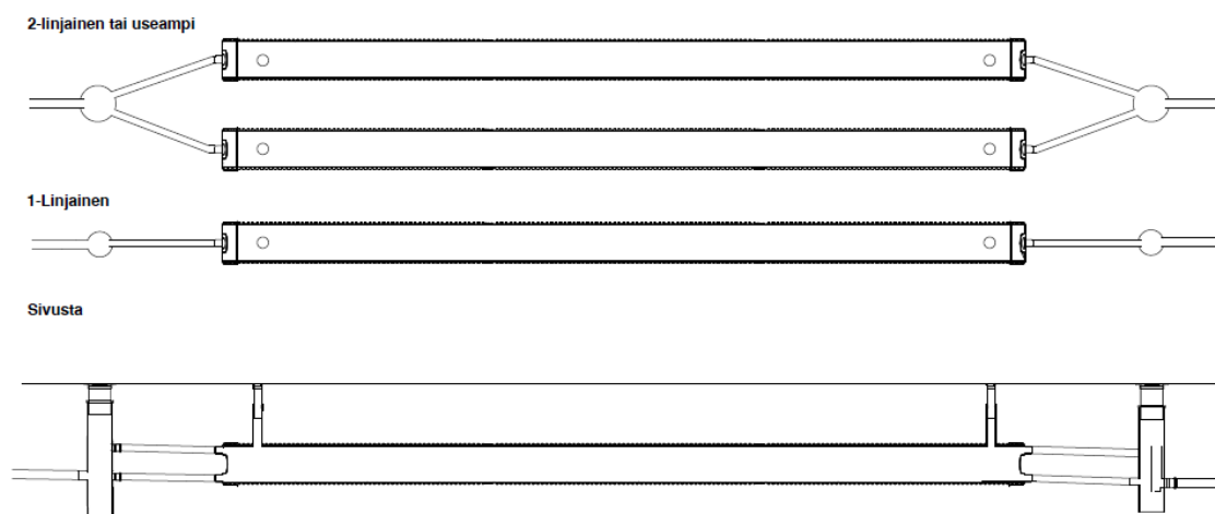
Kuva 1. Esimerkki 1- ja 2-linjaisesta viivytysjärjestelmästä.
