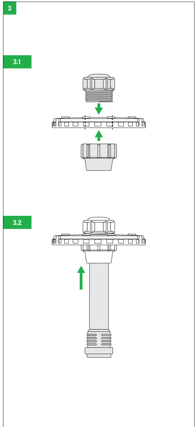
Kuva 3. Asenna päätihattu (5) reikään ja kiinnitä se sen kiristysmutterilla (4) niin, että muhvi osoittaa säiliön sisään päin (kuva 3.1). Paina suojaputki (3) päätihatun muhvin pohjaan asti (kuva 3.2).
