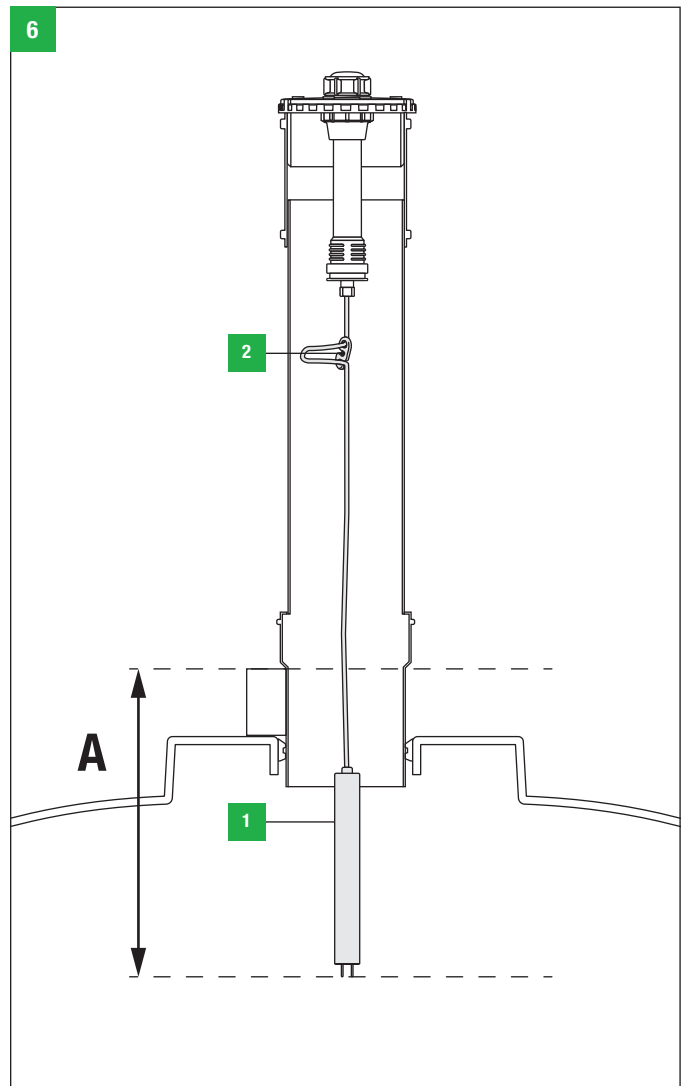
Kuva 6. Pinta-anturi (1) roikkuu kaapelistaan säiliössä. Kun nestepinta oikosulkee elektrodit, aktivoituu nestepinnan hälytys.
