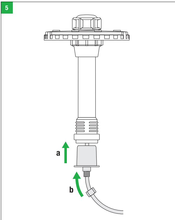
Kuva 5. Aseta piirikortti suojausputken (3) sisään. Vaihe a : paina päätytulppa (2) suojausputken (3) muhvin pohjaan asti. Vaihe b : kiristä kaapeliläpivienti (1).
