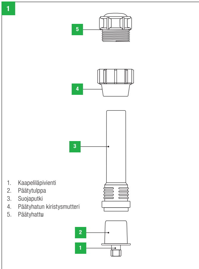
Kuva 1. Lähetinyksikön osat.
