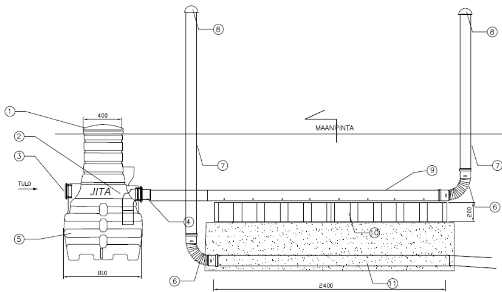
In-drän moduuli 2kpl+hiekkasuodatus 30cm
